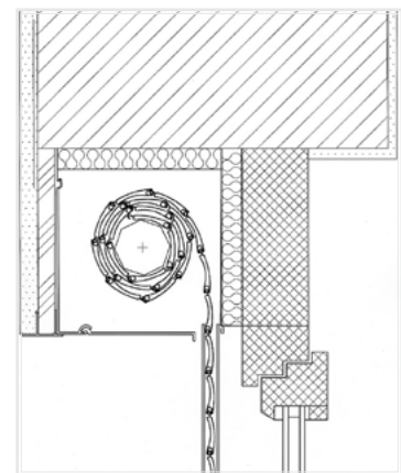
Skrzynka rolety wbudowana pod istniejące nadproże.
