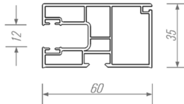
PG 01 - prowadnica moskitiery
