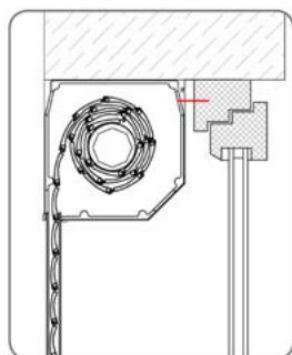
TYP „A” ROLETA ZAMONTOWANA WE WNĘCZE OKNA (PRAWOSKRĘTNA).
