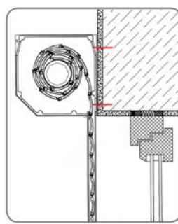
TYP „C” ROLETA ZAMONTOWANA NA ŚCIANIE BUDYNKU (LEWOSKRĘTNA).
