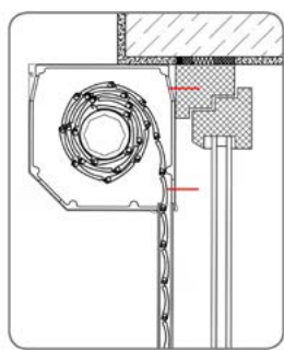
TYP „B” ROLETA ZAMONTOWANA WE WNĘCZE OKNA (LEWOSKRĘTNA).
